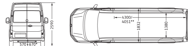
Crafter 35 Van LWO High Roof
